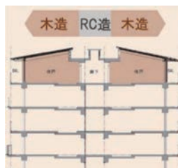
最上階構造図
